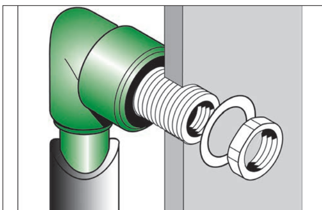
Переходной угольник aquatherm green pipe (внутренняя резьба/ наружная резьба) для полрых стен с резьбой длиной 30 мм.
