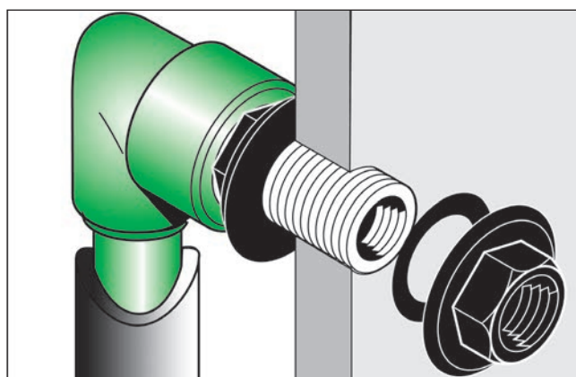
Деталь aquatherm green pipe для подключения к полрой стене с переходным угольником aquatherm green pipe.
