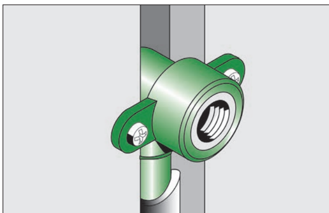
Настенная шайба aquatherm green pipe для полрой стены устанавливается в канале стены.
