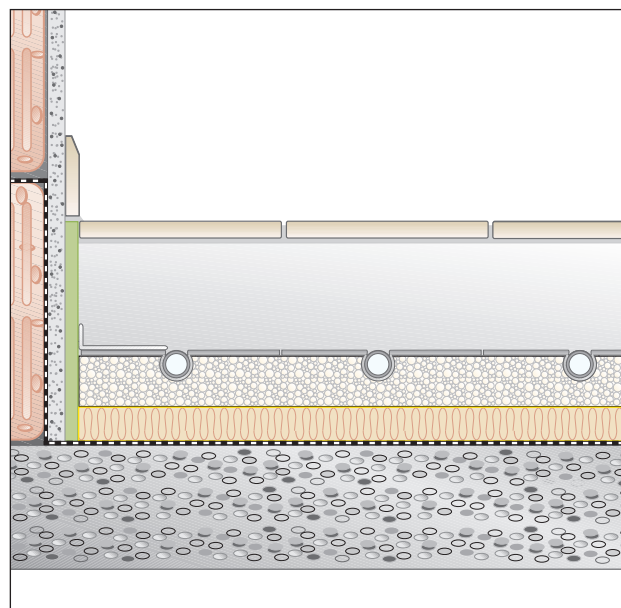
системный элемент TS 30 перекрытия, граничащие с грунтом
