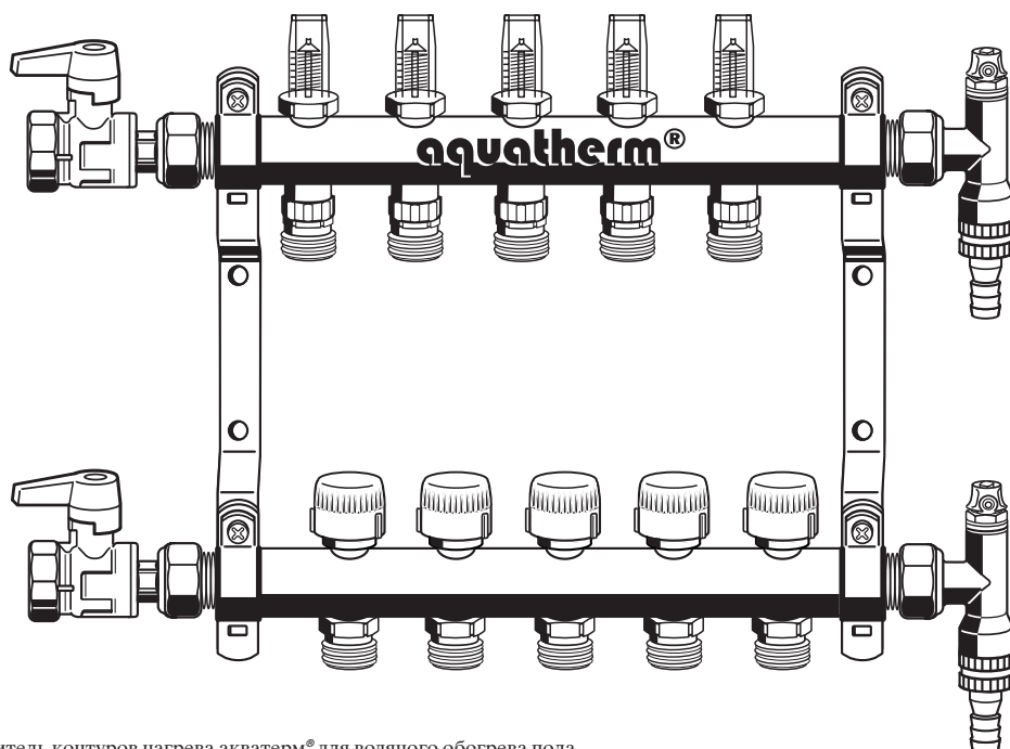
распределитель контуров нагрева акватерм® для водяного обогрева пола
