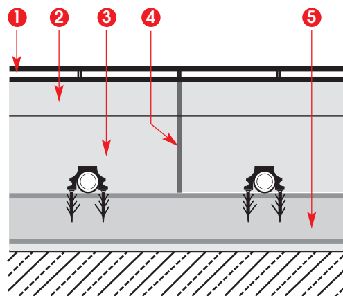
правильное распределение деформационных швов
