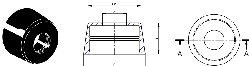
aquatherm red pipe - Крышка соединительного элемента для спринклера с открытой установкой
