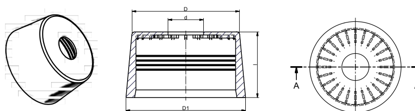
aquatherm red pipe - Крышка соединительного элемента для спринклера со скрытой установкой
